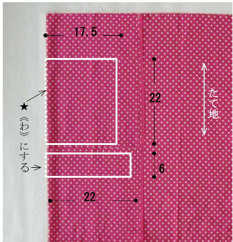
リボンゴム布 《わ》にして1枚
